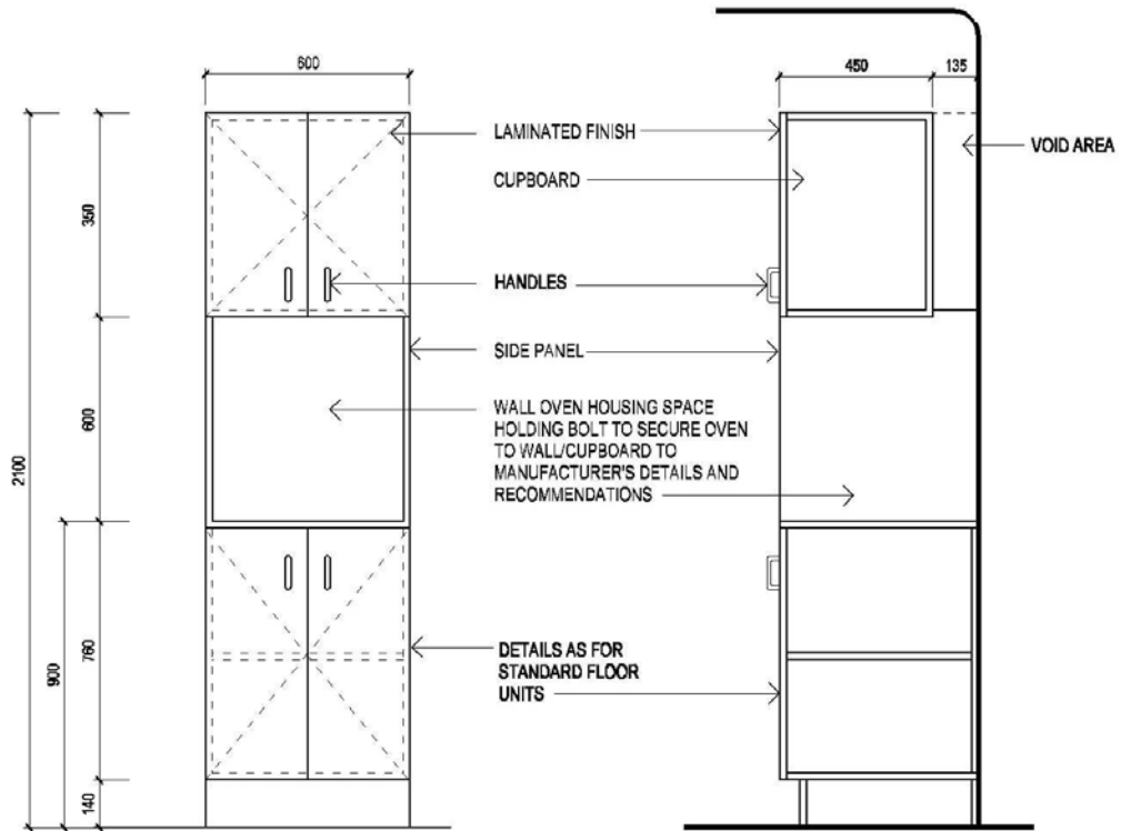
ELEVATION
